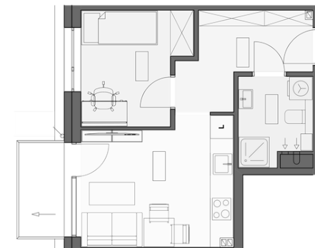
RZUT 2D
